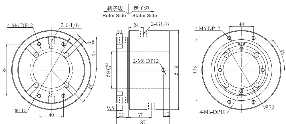
3602006 (2进2出, 6~8mm气管, 孔径60mm, 纯气动旋转接头) 尺寸图
